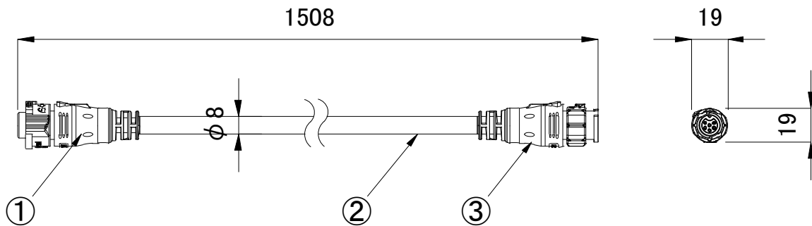
専用ジャンパーケーブル 5ft (1.5m)
