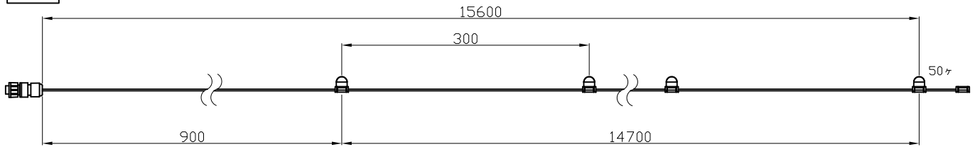
全体図
