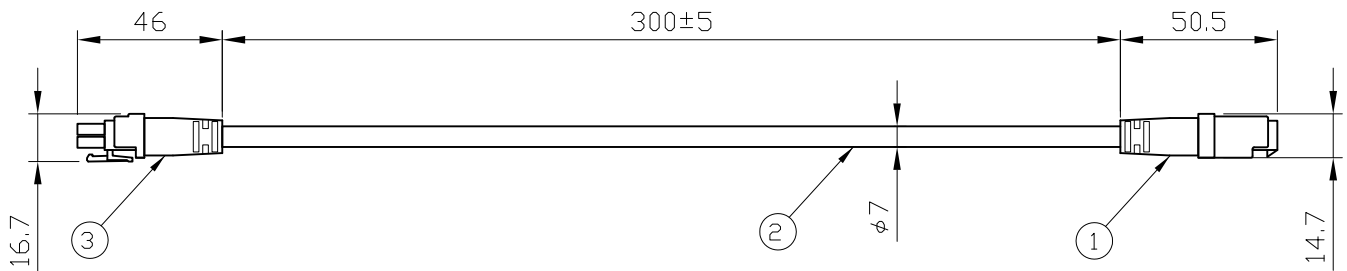
eW Cove Powercore専用ジャンパーケーブル 1フィート(0.3m)
