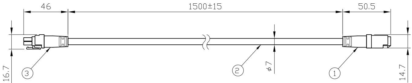
eW Cove Powercore専用ジャンパーケーブル 5フィート(1.5m)
